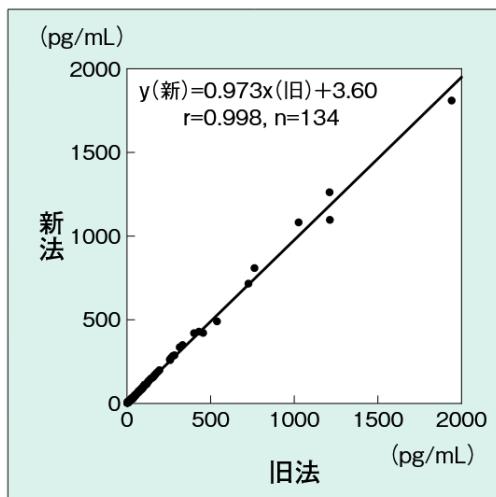
ACTH相関
